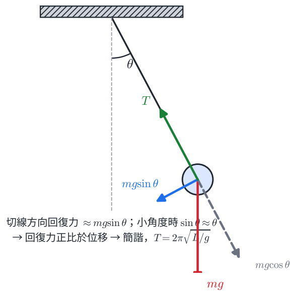
圖 5-4：單擺受力分解。重力沿擺線的分量 mg \cos \theta 與張力相關，沿切線的分量 mg \sin \theta 指向平衡位置，即為回復力；小角度時 \sin \theta \approx \theta ，回復力近似正比於位移，故近似為簡諧。
